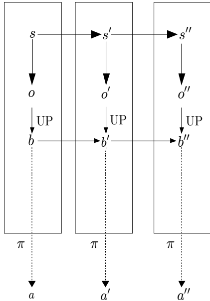
Figure 1.8: Représentation détaillée d'un POMDP
