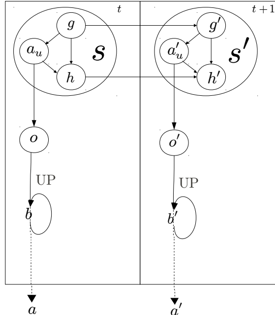
Figure 1.14: Diagramme d'influence d'un POMDP dont l'état est décomposé en trois composants : but, action utilisateur et historique.
