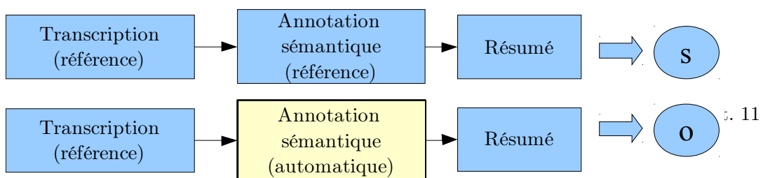
Figure 3.2 : Système « SLU », sans erreur de reconnaissance (annotation de référence pour l'ASR) et avec erreur de compréhension SLU.
