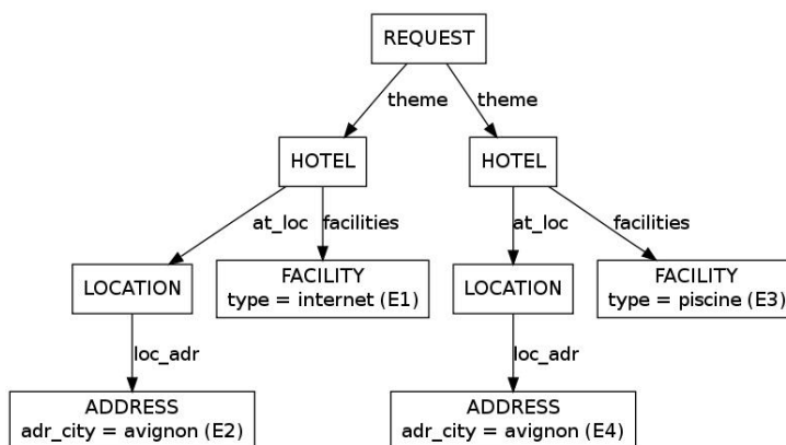
Figure 2.2 : État de dialogue permettant de générer plusieurs requêtes.
